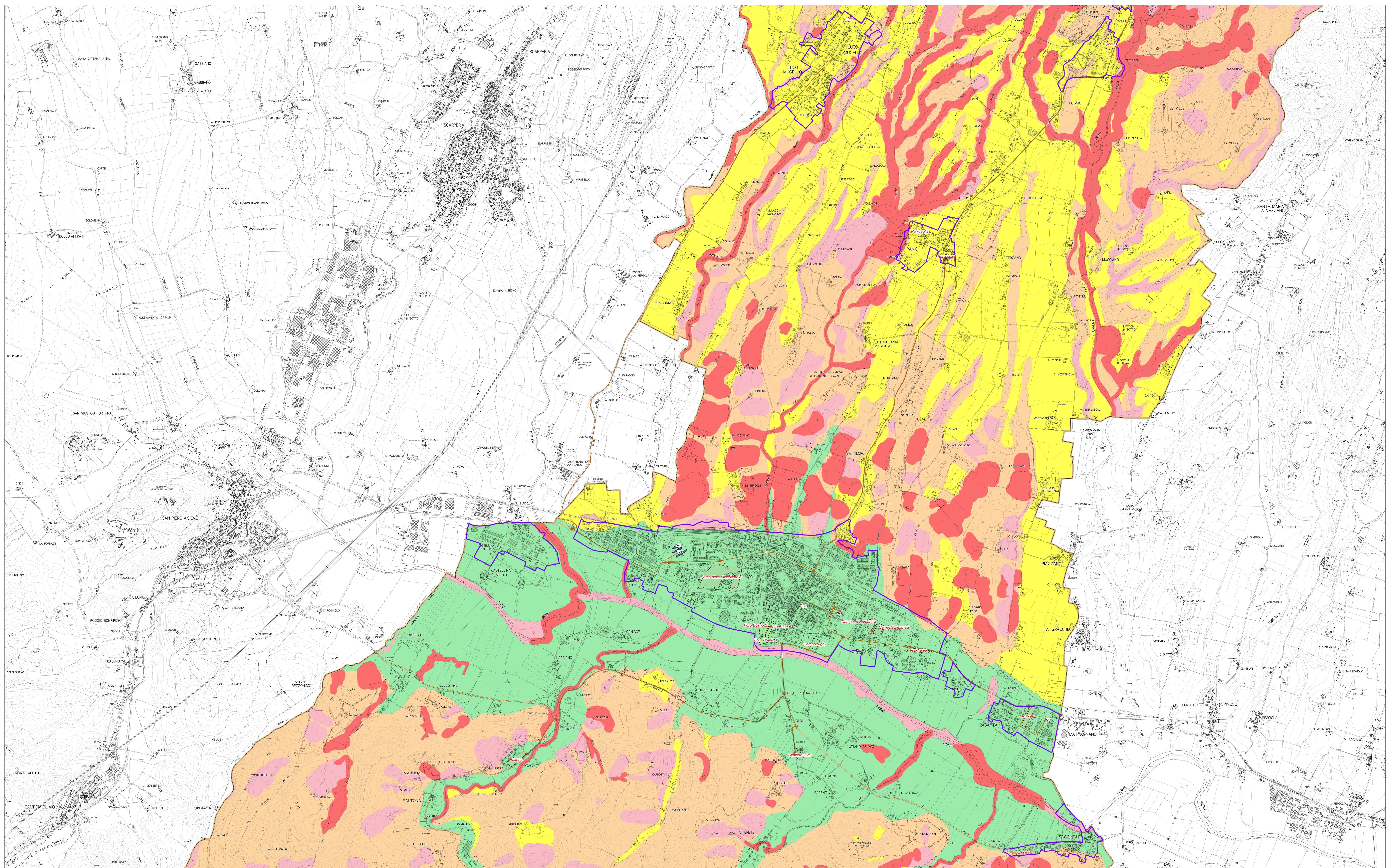
GEO01.2 - Carta delle aree ed elementi esposti a fenomeni geologici
