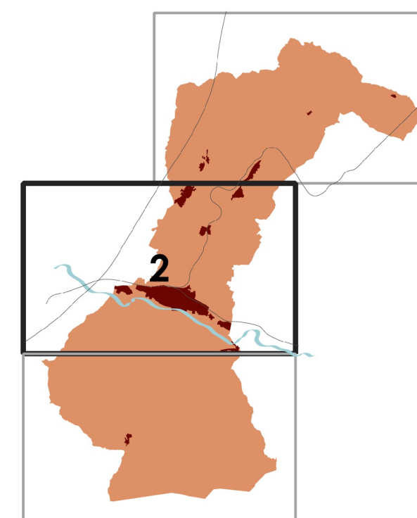
GEO01.2 - Carta delle aree ed elementi esposti a fenomeni geologici
